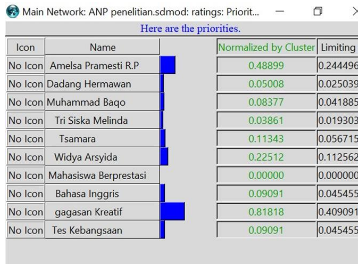
Gambar 5. Hasil Akhir Perhitungan menggunakan ANP
